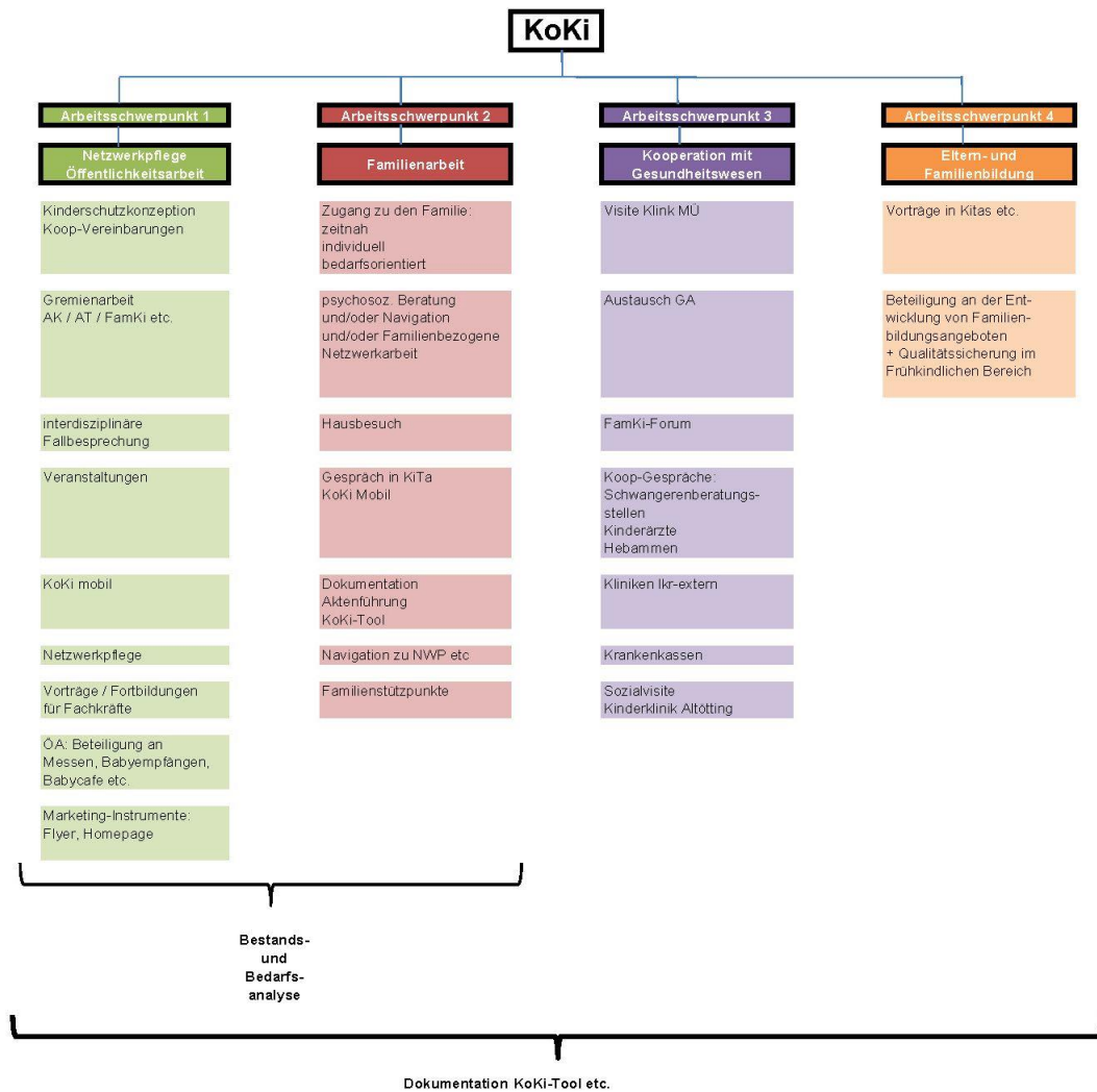
Abbildung 2: Arbeitsschwerpunkte
